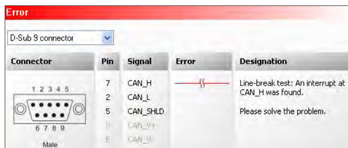
Wiring test
